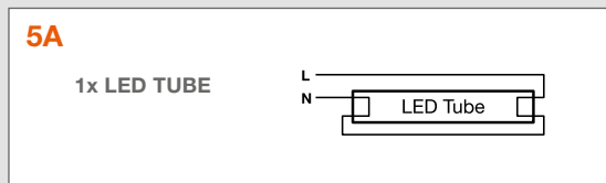
Herbedrading volgens bedradingsschema voor enkellamps armaturen
